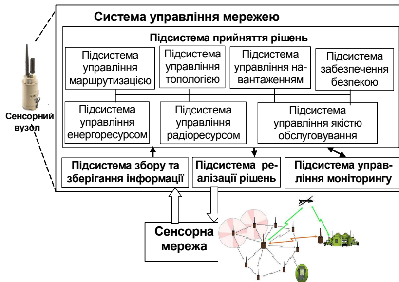
Рис. 5. Функціональна модель системи оперативного управління
