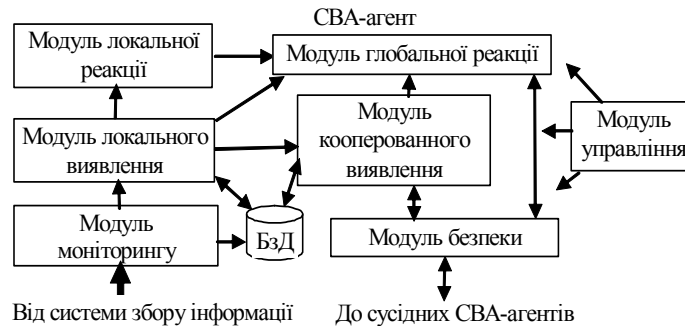
Рис. 11. Концептуальна модель IDS-агента
