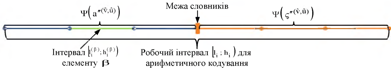
Рис. 3. Приклад побудови робочого інтервалу для арифметичного кодування
