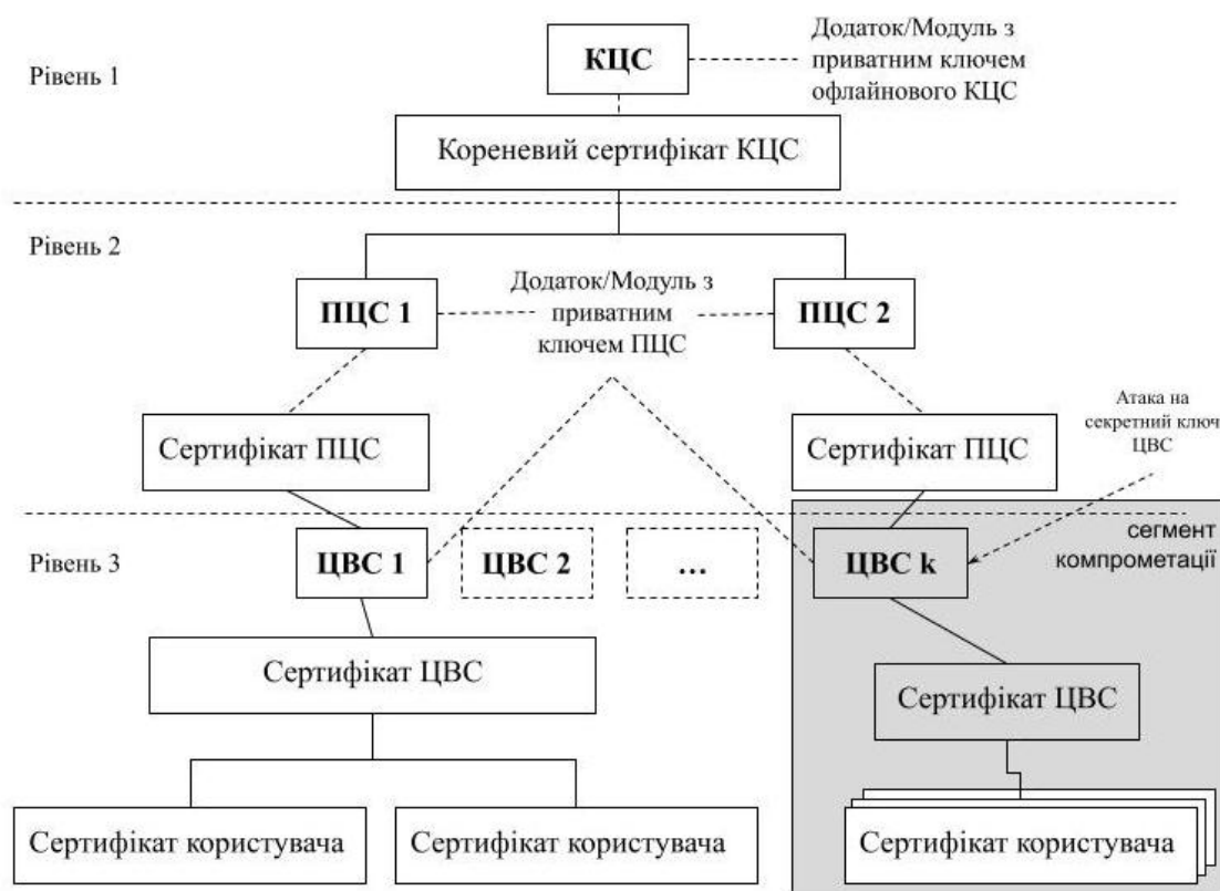
Рис. 3. Базова трирівнева архітектура PKI
