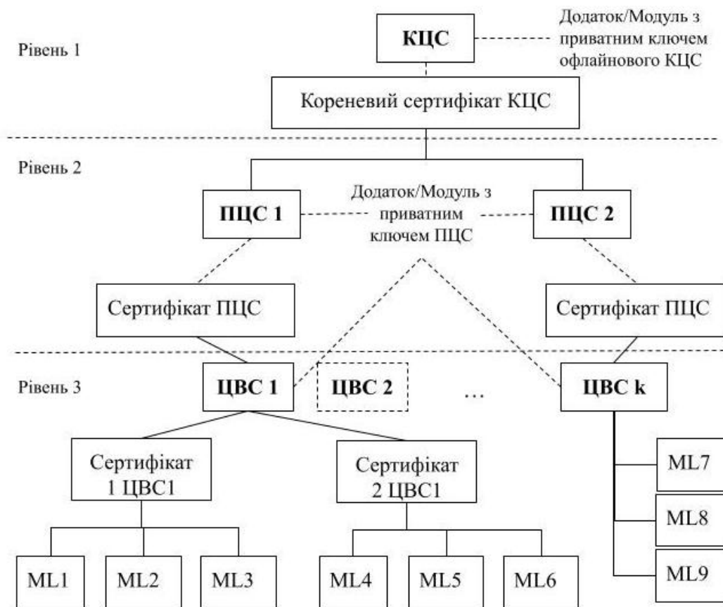
Рис. 7. Варіант альтернативної інфраструктури РКІ з використанням концепції DKMS та технології DMLT
