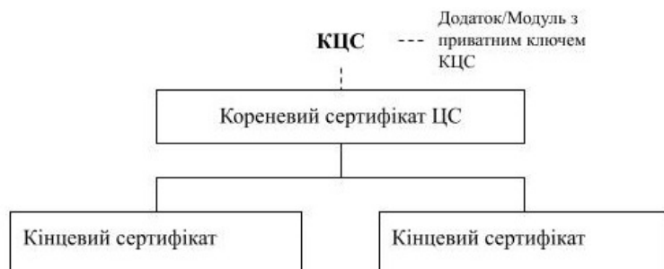
Рис. 1. Базова однорівнева архітектура РКІ
