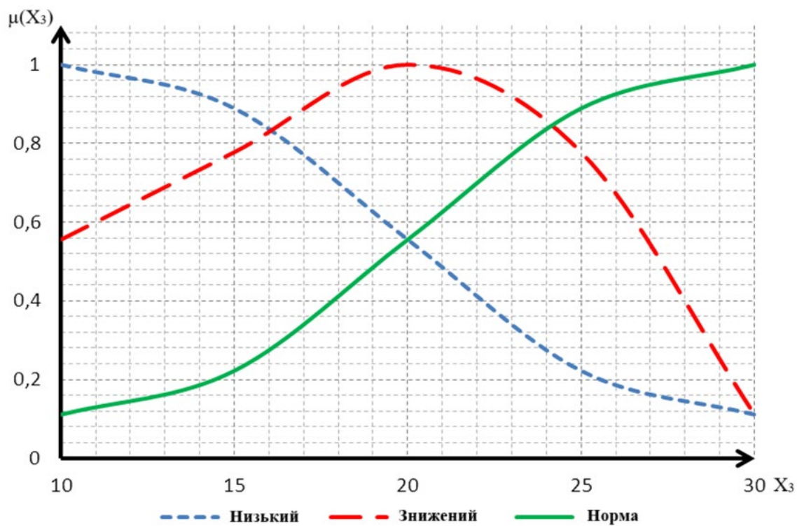
Рис. 5. Нечіткі множини параметра X_3
